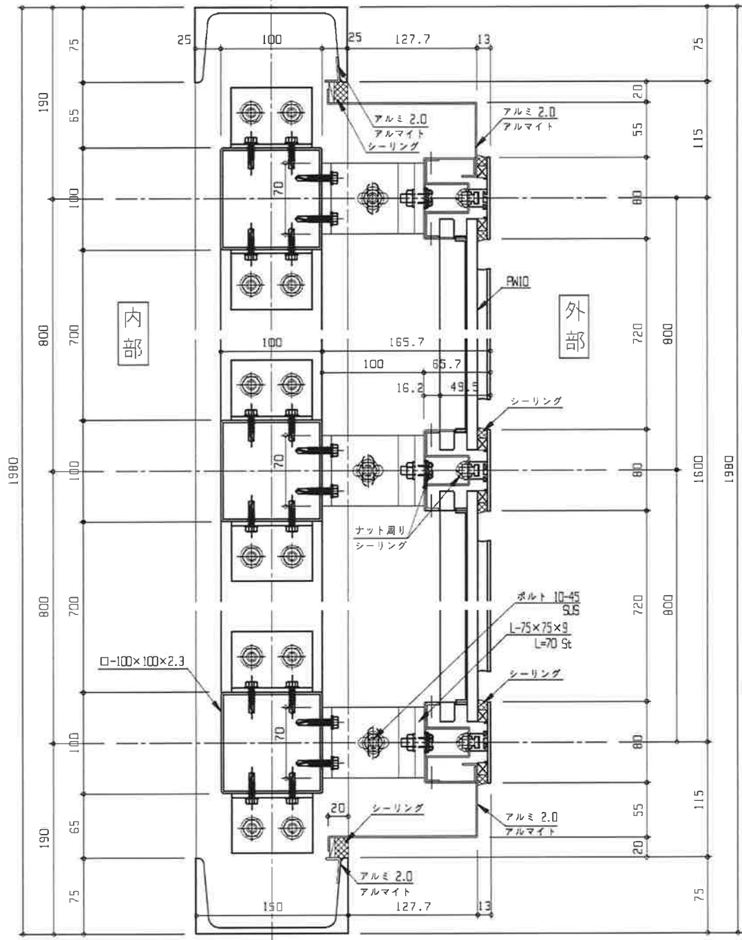
図-3 水平断面図
