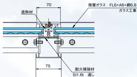
L方向断面図
