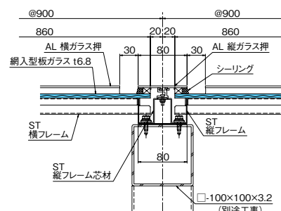
縦フレーム断面図
