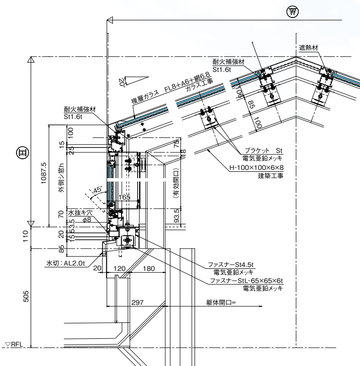
W方向断面図
