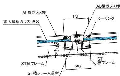
ガラスジョイント部断面図
