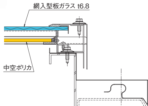
■ 横断面図
