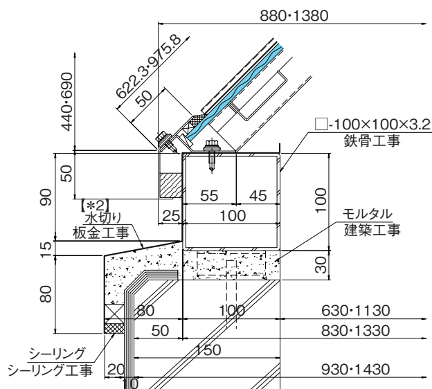
■ 横断面図
