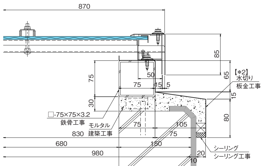
■ 横断面図
