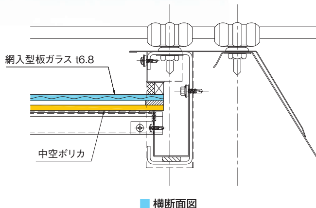
■ 横断面図
