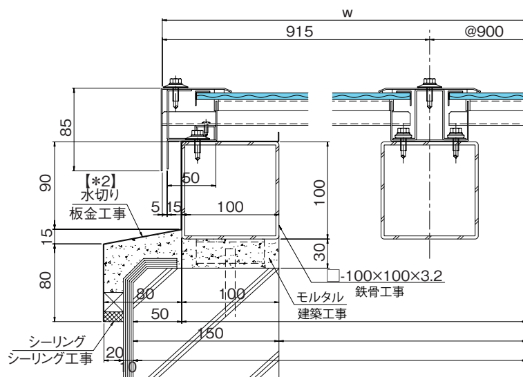
■ 横断面図
