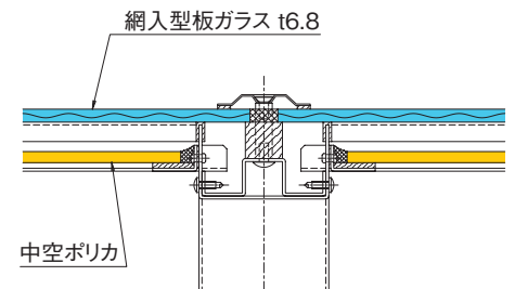
■ 横断面図
