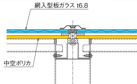
■ 横断面図
