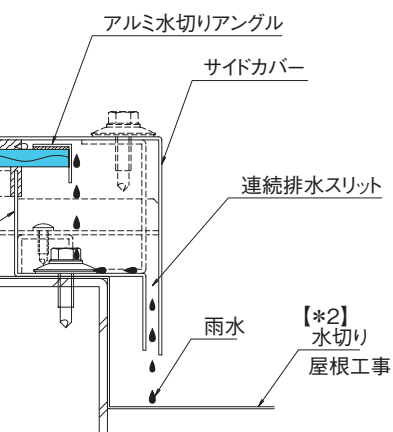
排水経路
