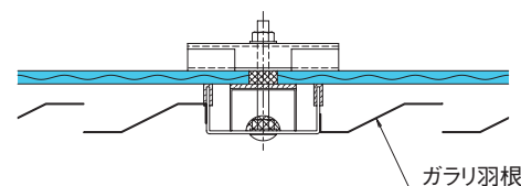
■ 横断面図
