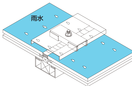
・単板ガラス + 中空ポリカ・複層ガラス ピースガラス押 + 目地保護カバー
