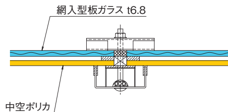
■ 横断面図
