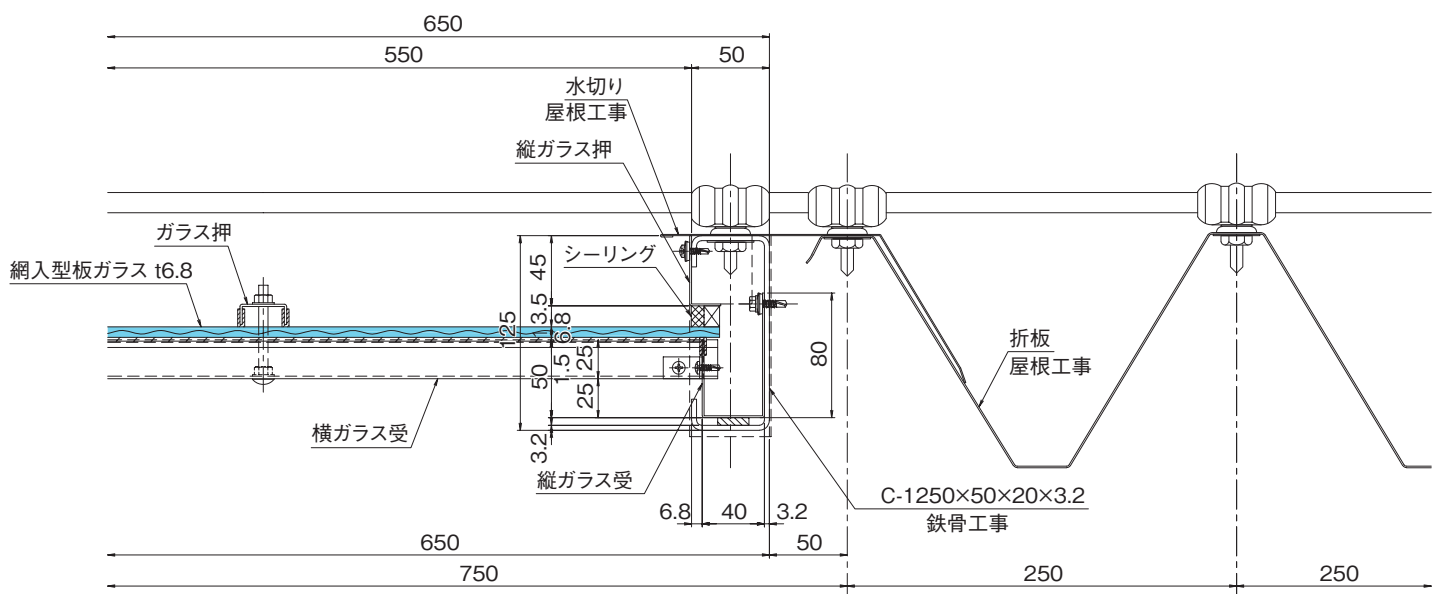
横断面詳細図
