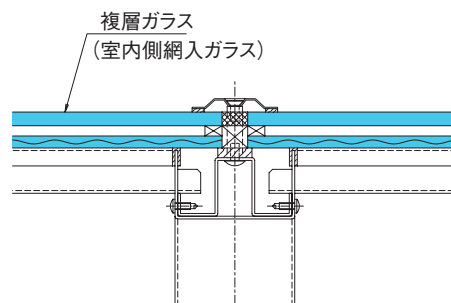
■ 横断面図
