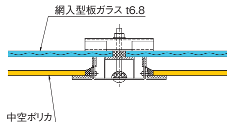
■ 横断面図
