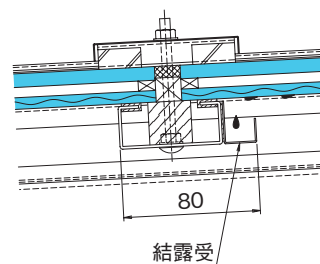
■ ジョイントガラス受断面図
