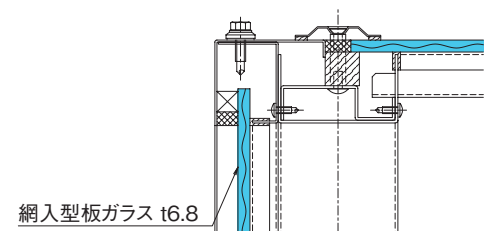
■ 横断面図
