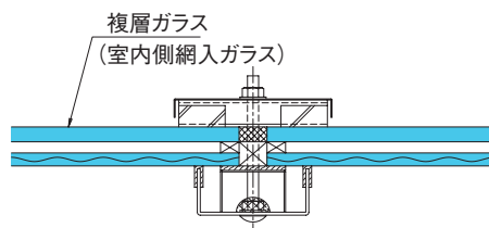
■ 横断面図
